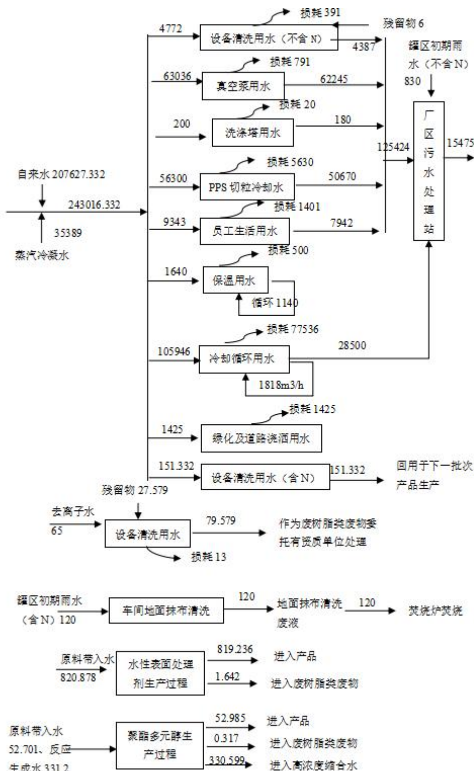
图 3.3-1 现有项目全厂水平衡图 (m³/a)
