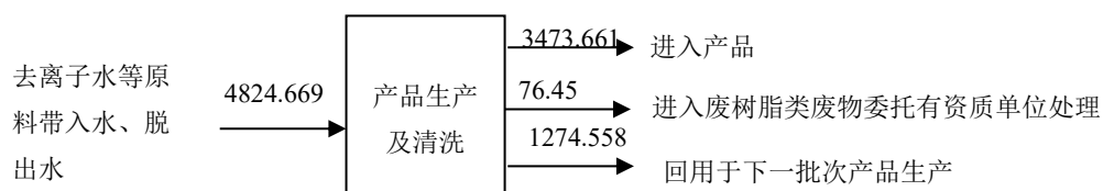
图 4.4-1 本项目水平衡示意图 (单位: t/a)
