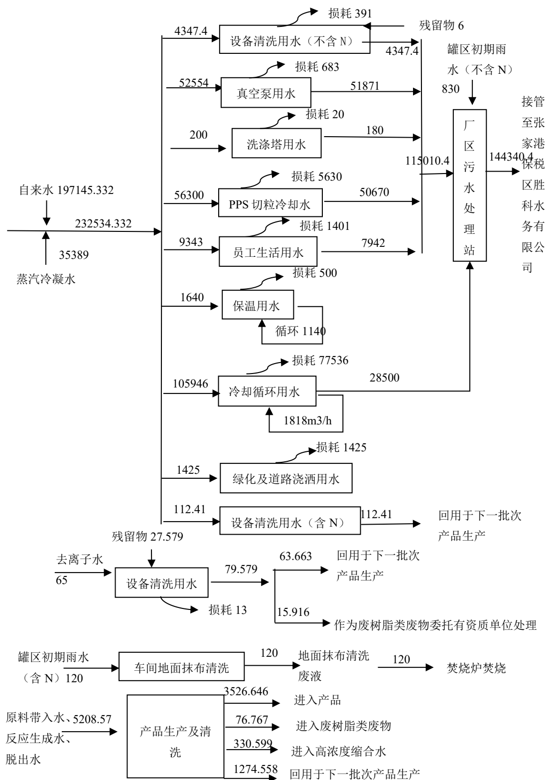
图 4.4-2 技改后全厂水平衡示意图 (单位: t/a)
