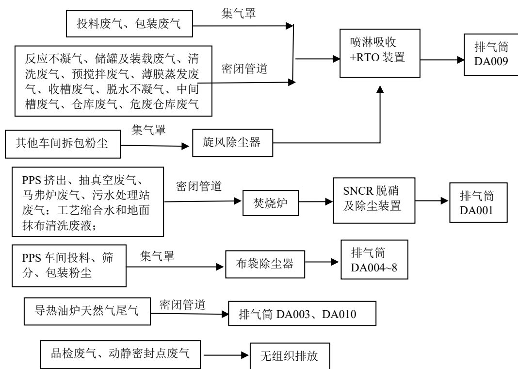
图 3.5-1 现有项目废气收集、处理工艺示意图
