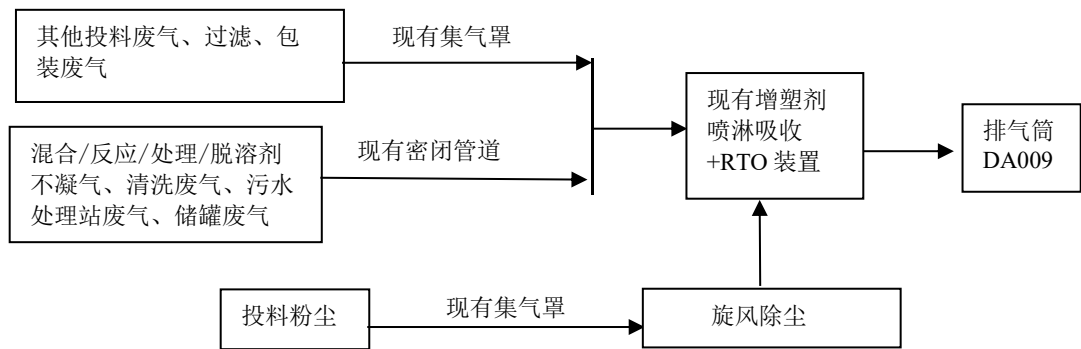
图 7.1-1 本项目废气收集处理工艺流程图
