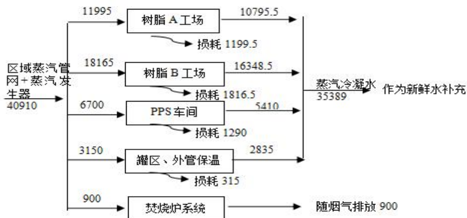
图 4.4-3 技改后全厂蒸汽平衡示意图 (单位: t/a)
