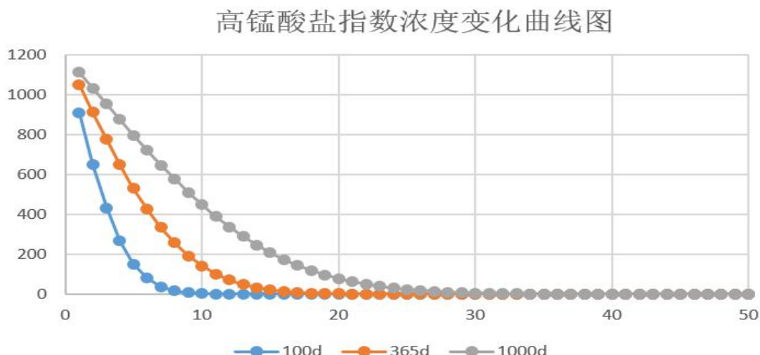
图 6.5-1 CODMn 浓度迁移变化预测图
