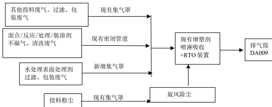
图 7.1-1 本项目废气收集处理工艺流程图
