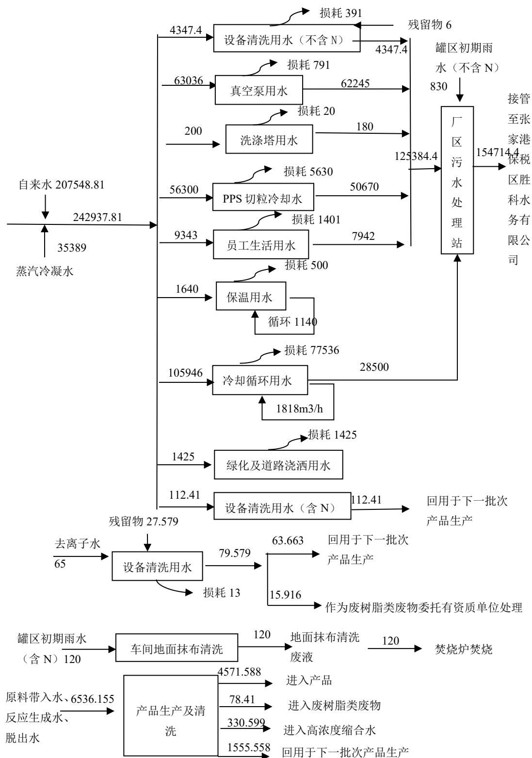
图 4.4-2 技改后全厂水平衡示意图 (单位: t/a)
