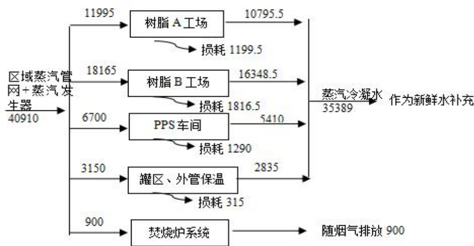
图 3.3-2 现有项目全厂蒸汽平衡图
