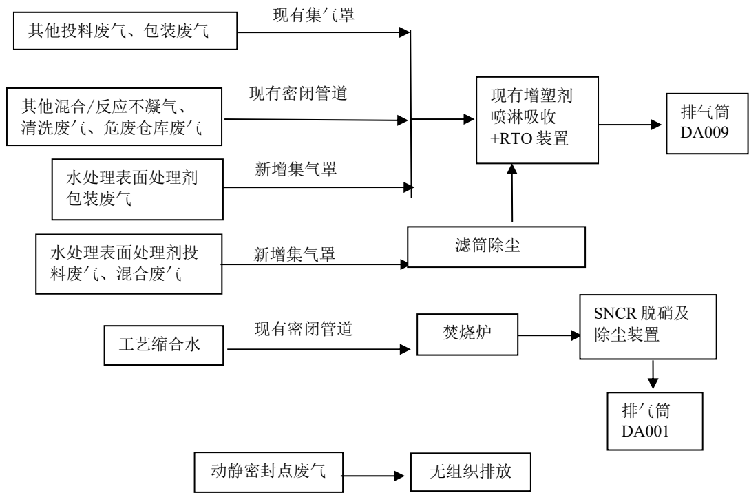
图 7.1-1 本项目废气收集处理工艺流程图
