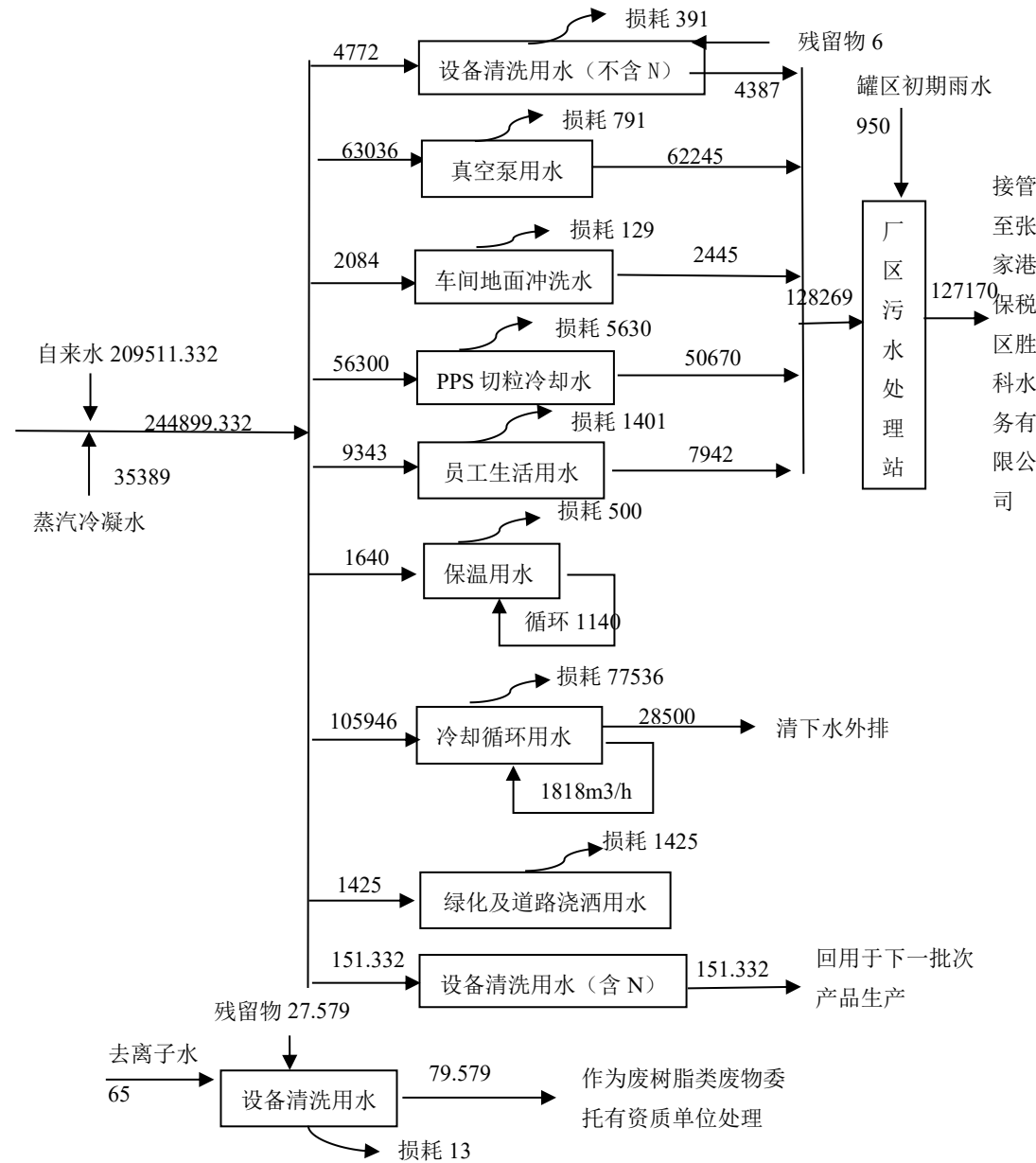
图 4.4-10 扩建后全厂水平衡示意图（单位：t/a）
