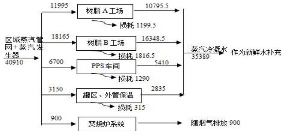
图 4.4-10 扩建后全厂水平衡示意图（单位：t/a）
