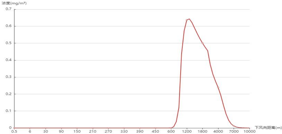
图 6.7-3 火灾 CO（最不利气象条件）下风向浓度变化图
