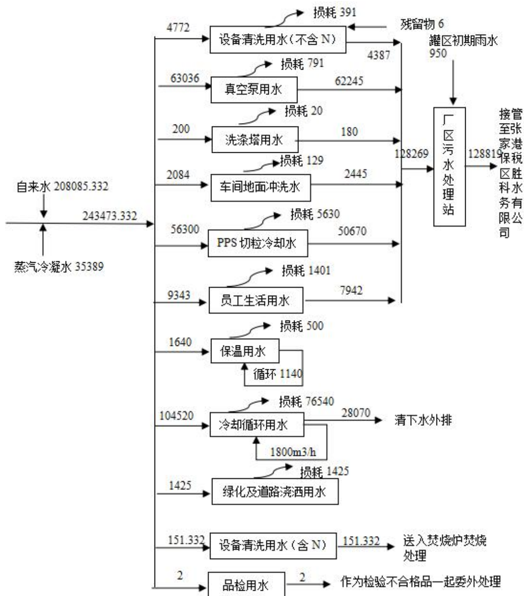
图 3.3-1 现有项目全厂水平衡图 ( \text{m}^3/\text{a} )
