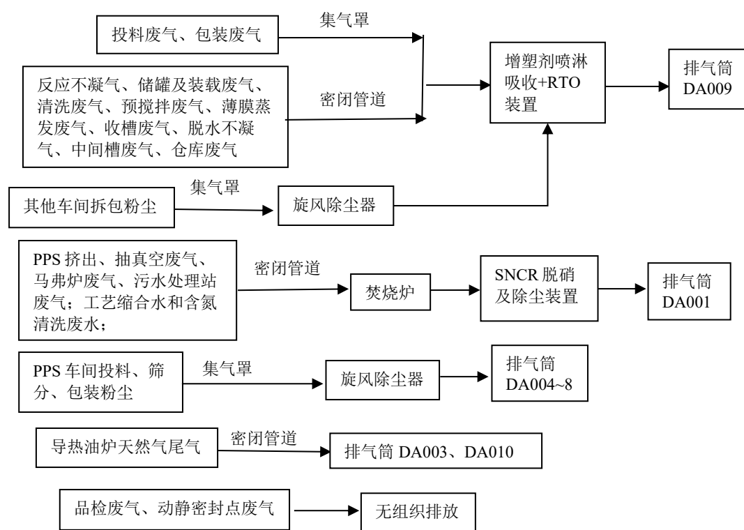
图 3.5-1 现有项目废气收集、处理工艺示意图
