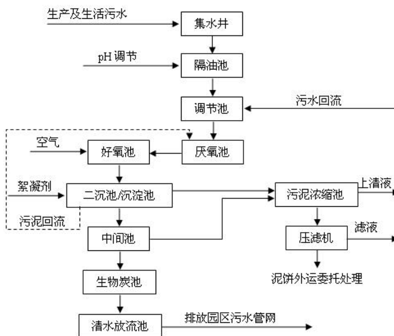
图 3.5-2 废水预处理工艺流程图
