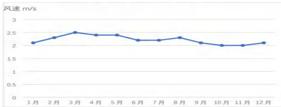
图 6.1-2 平均风速的月变化曲线
