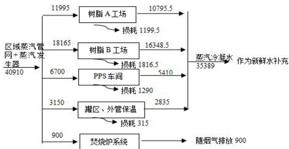
图 3.3-2 现有项目全厂蒸汽平衡图
